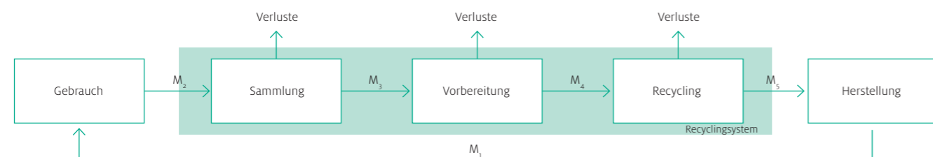
Abbildung 1: Vereinfachtes Entsorgungssystem, in dem M_1 bis M_5 Gesamtmassenflüsse an einer bestimmten Stelle der Verarbeitungskette darstellen. «Vorbereitung» entspricht allen manuellen und mechanischen Verarbeitungsprozessen, welche Endfraktionen für die letzten Behandlungsschritte, das Recycling, erzeugen.
